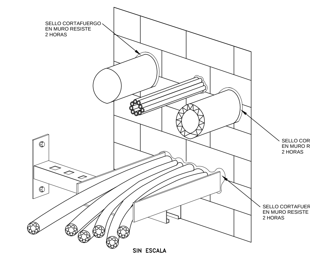
DETALLE CORTAFUEGO EN PASANTES HORIZONTALES SIN ESCALA
