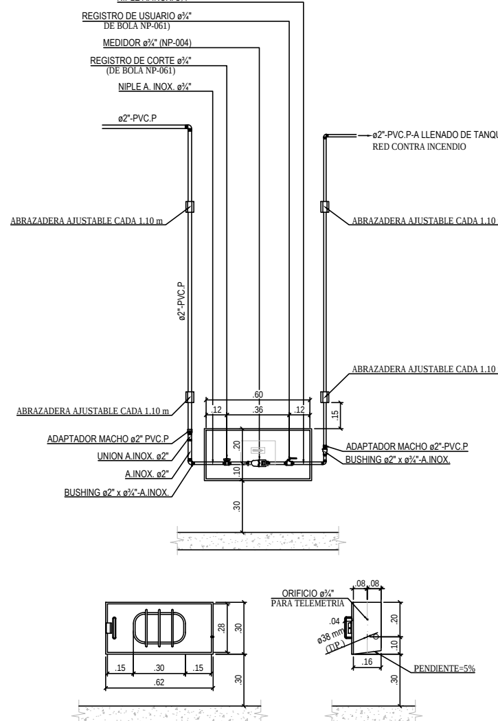
DETALLE CAJILLA 1 MEDIDORES Ø½" AGUA FRIA POTABLE SIN ESCALA
