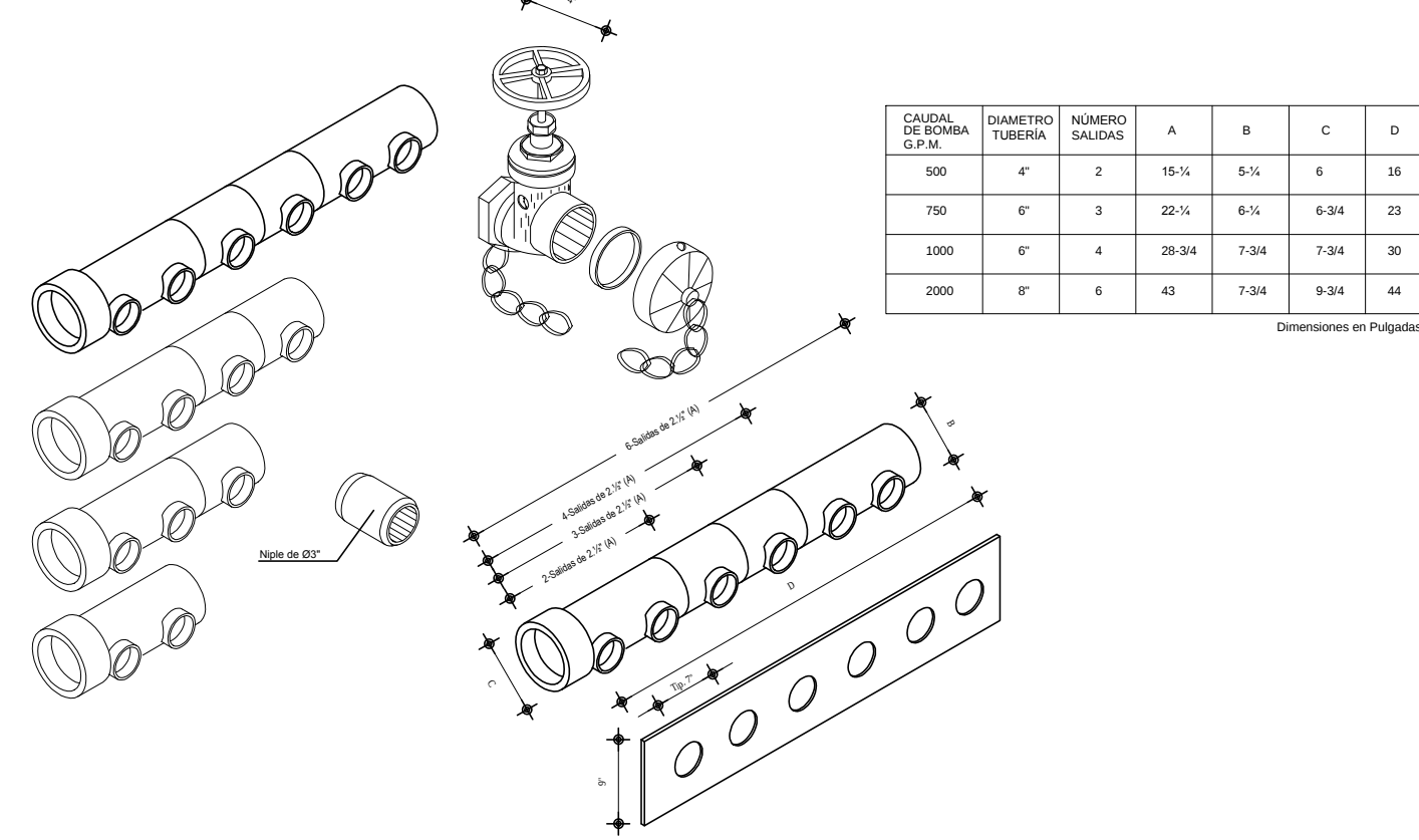
DETALLE CABEZAL DE PRUEBA SIN ESCALA
