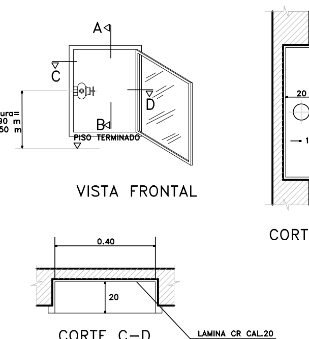
DETALLE CONEXION DE MANGUERA CLASE I CON CAJA DE PROTECCION SIN ESCALA
