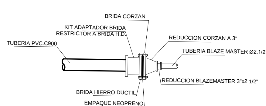
DETALLE DE TRANSICION PVC.C900 – BLAZE MASTER EN LAS REDES DE INCENDIO
