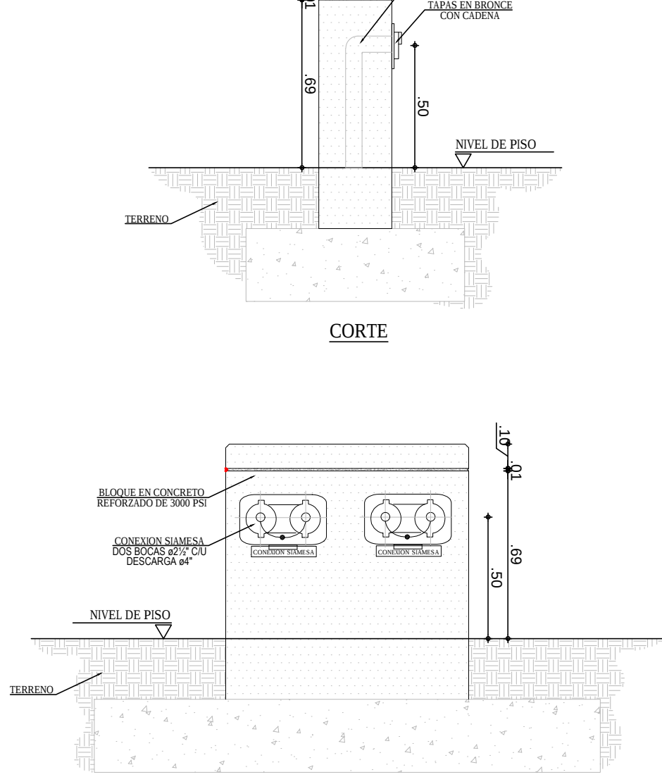
DETALLE SIAMESA SIN ESCALA
