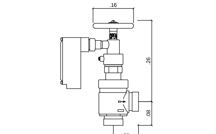
DETALLE VALVULA REDUCTORA DE PRESION. LISTADA PARA USO COMO VLV. VALVULA DE CONTROL INDICADORA Y VALVULA CHEQUE SIN ESCALA
