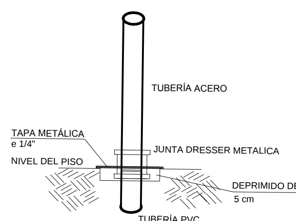
DETALLE DE TRANSICION PVC – ACERO EN LAS REDES DE INCENDIO
