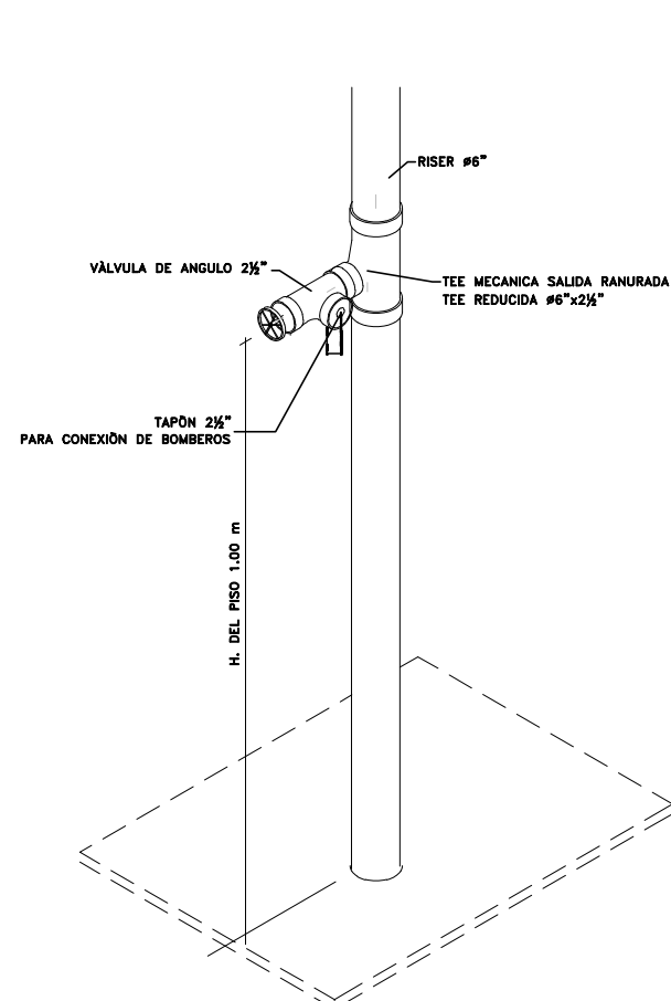
DETALLE SISTEMA CONEXION DE MANGUERA CLASE 1 Ø2½" SIN ESCALA
