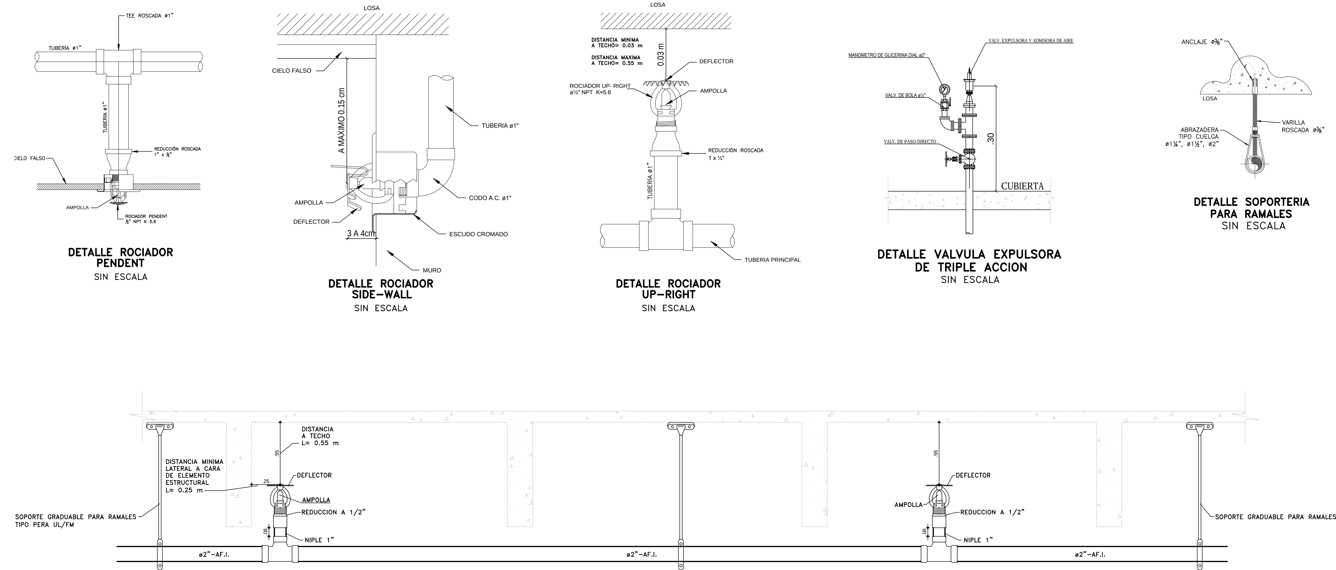
DETALLE INSTALACION ROCIADOR TIPO UP-RIGHT DE PISO 2 A PISO 11 SIN ESCALA
