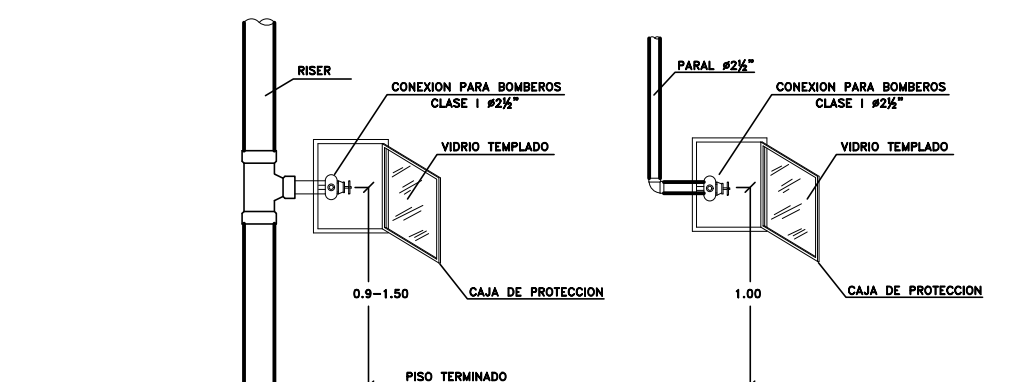
CONEXION DE MANGUERA CLASE I OPCION CON CAJA DE PROTECCION SIN ESCALA
